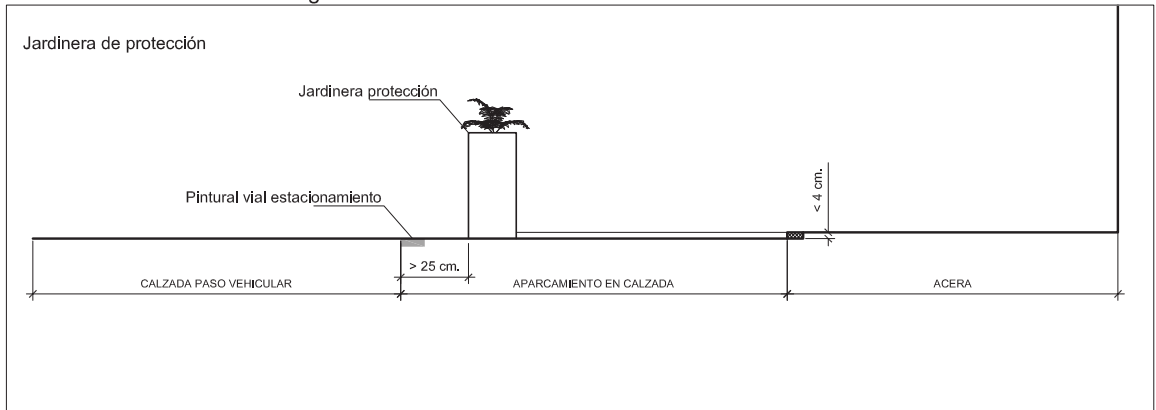
Velador en calzada: Detalles fig. 4
