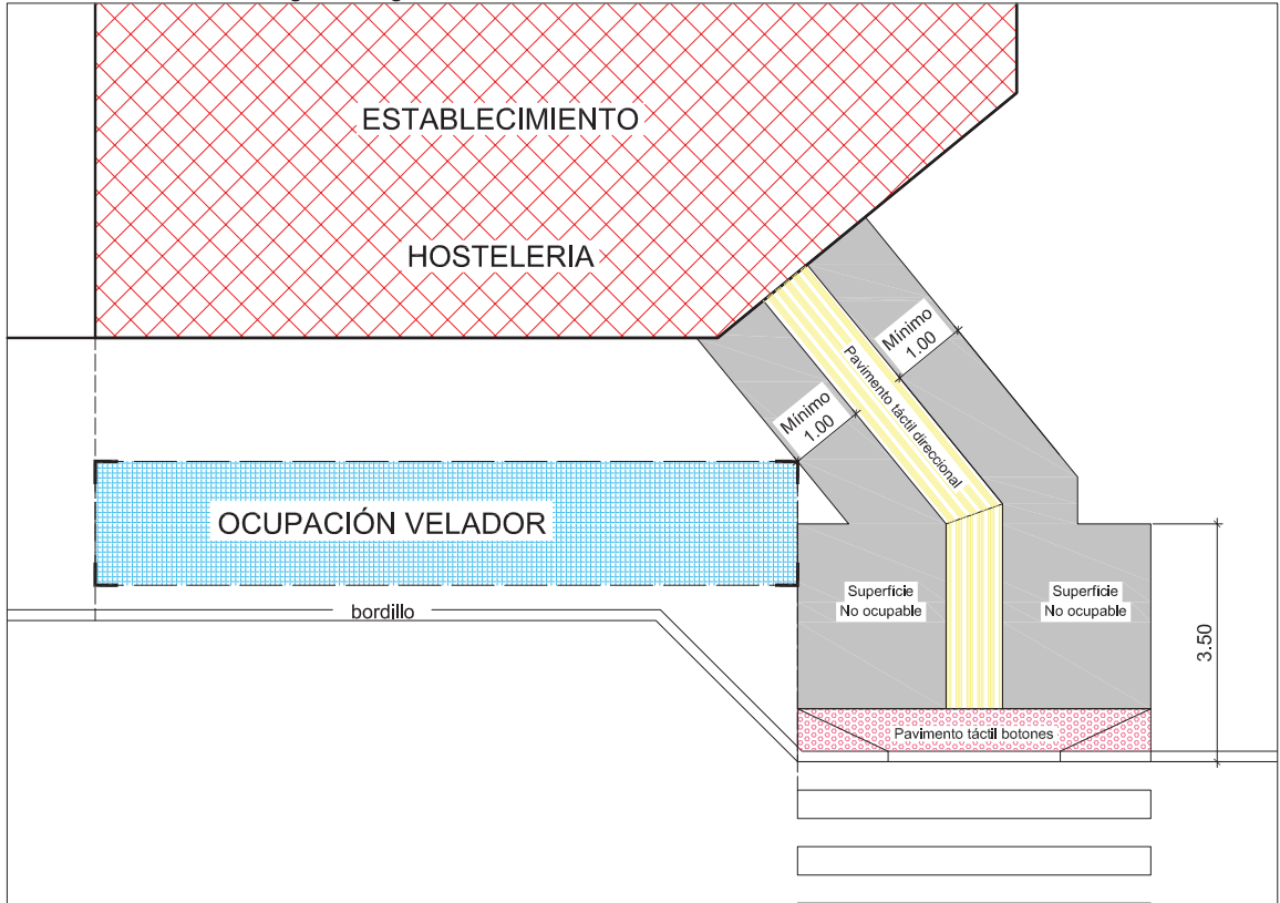
Distancias mínimas de seguridad fig. 1
