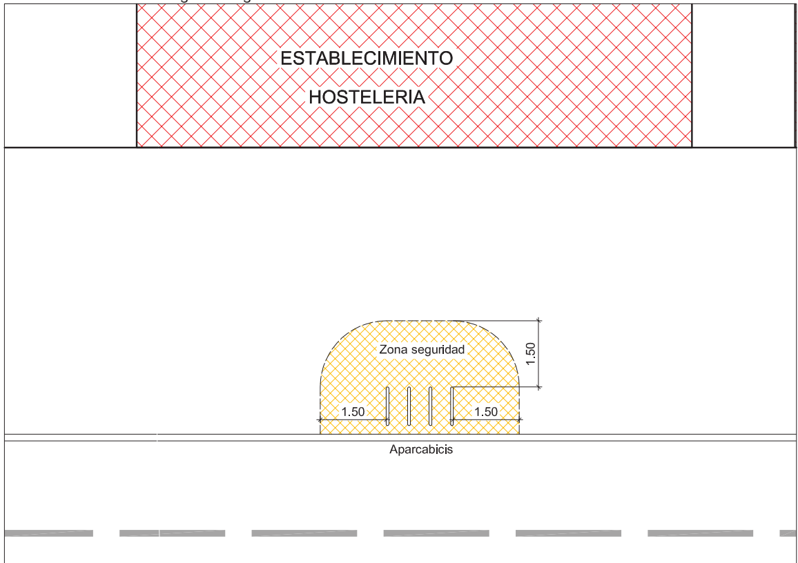
Distancias mínimas de seguridad fig. 4
