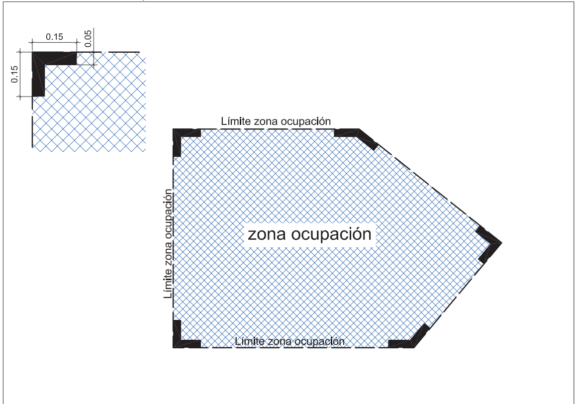
Velador : marcado zona ocupación
