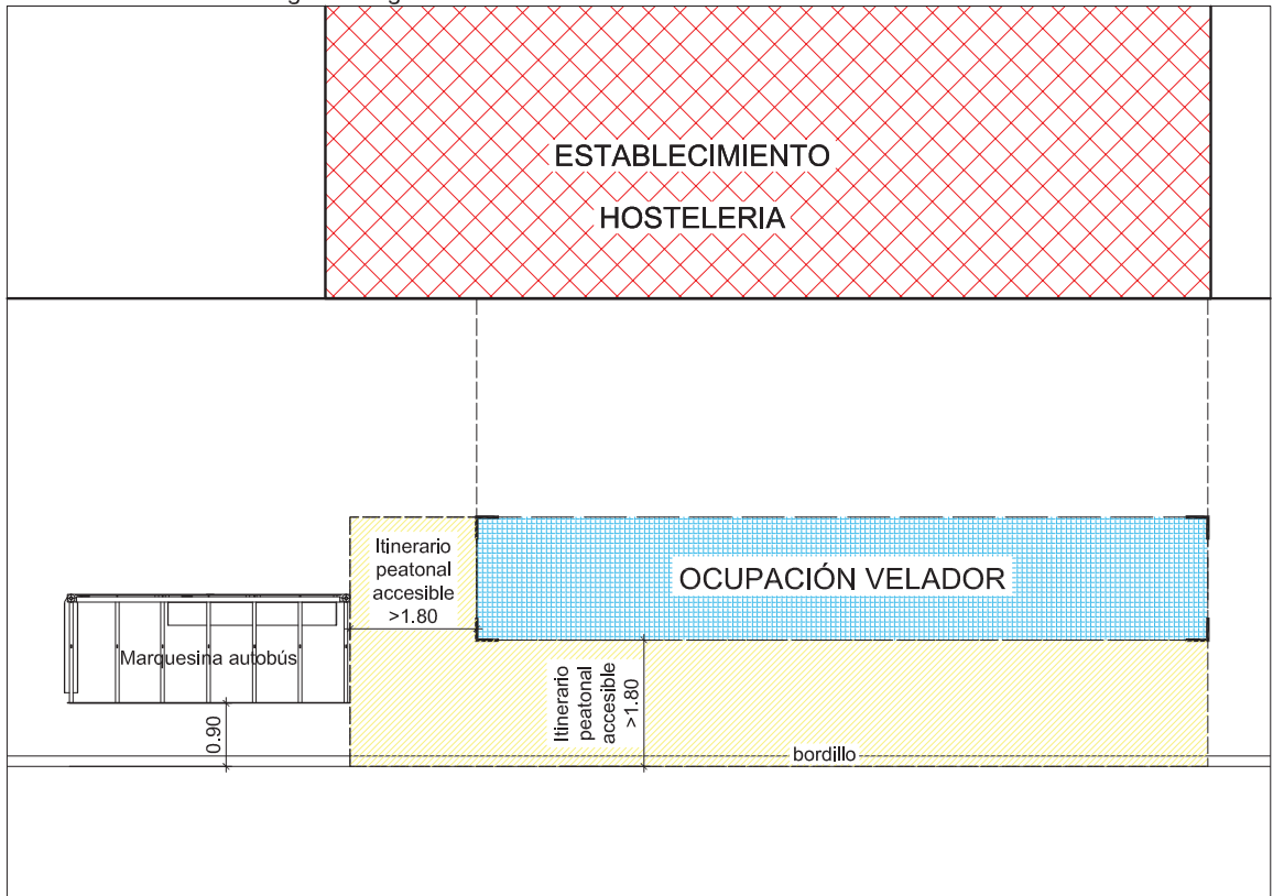
Distancias mínimas de seguridad fig. 2
