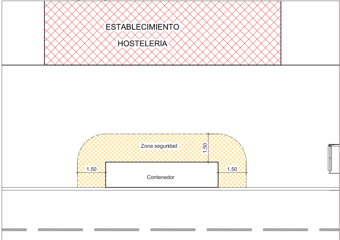
Distancias mínimas de seguridad fig. 3
