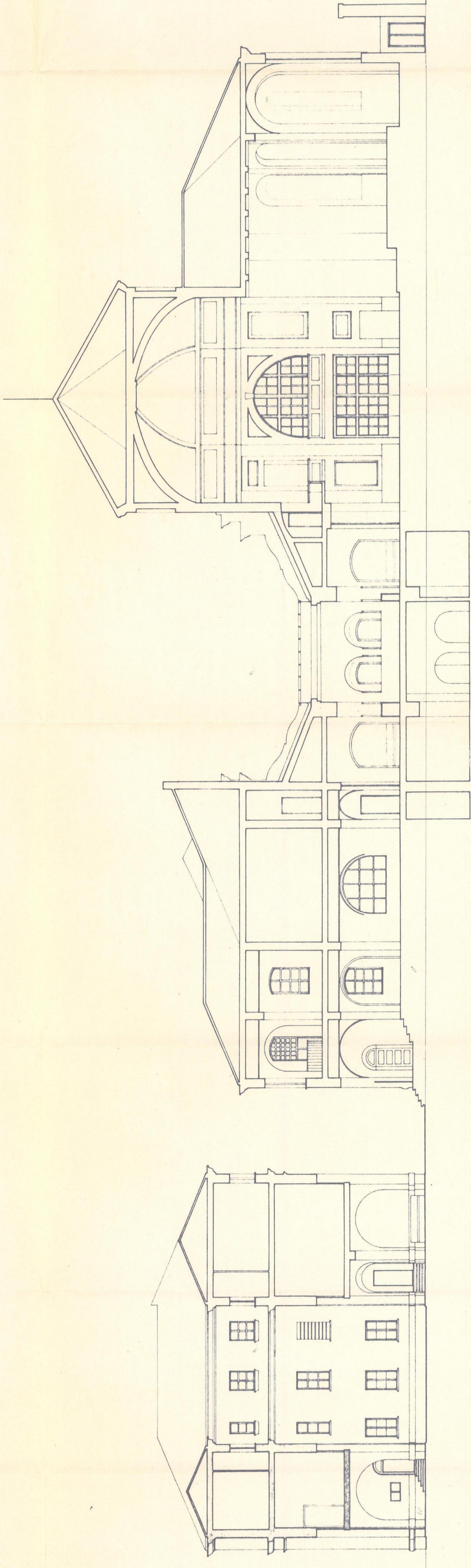
SECCION 1-1
