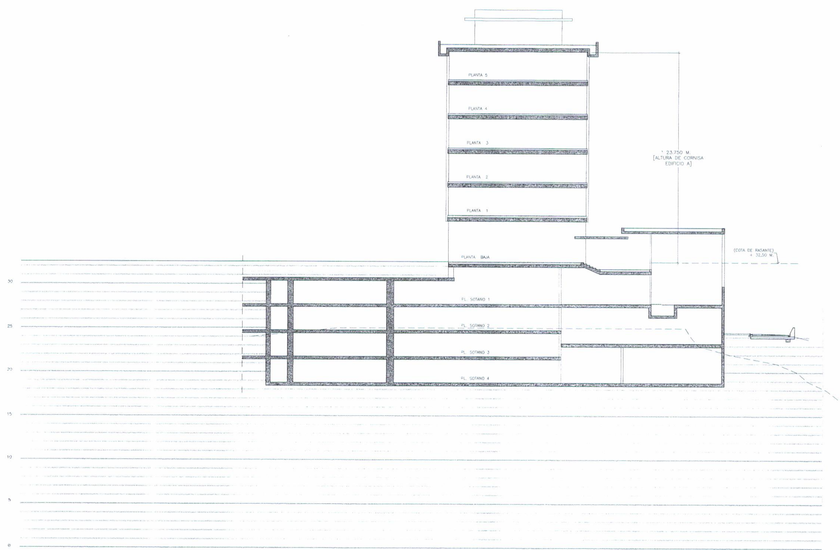
SECCION FASE 2
