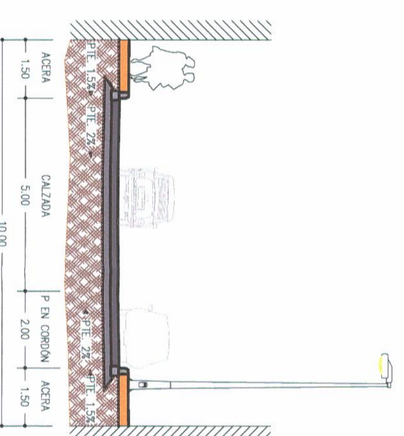
SECCIÓN CALLE 10 m VISTAHERMOSA-ORGEGIA
