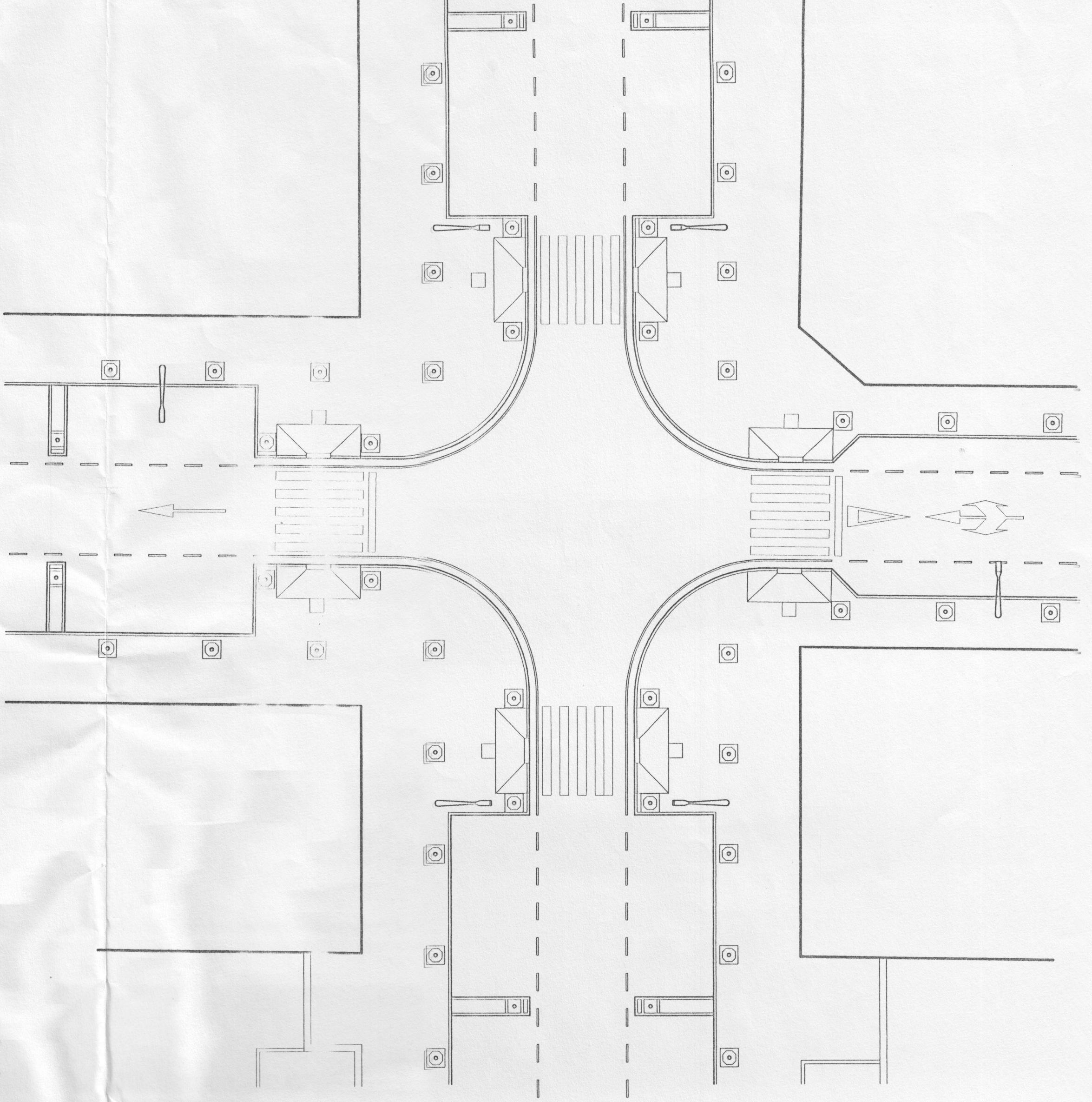
DETALLE CRUCE TIPO 1 ESCALA 1/200
