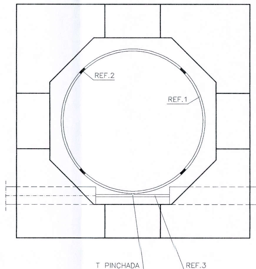
PLANTA
