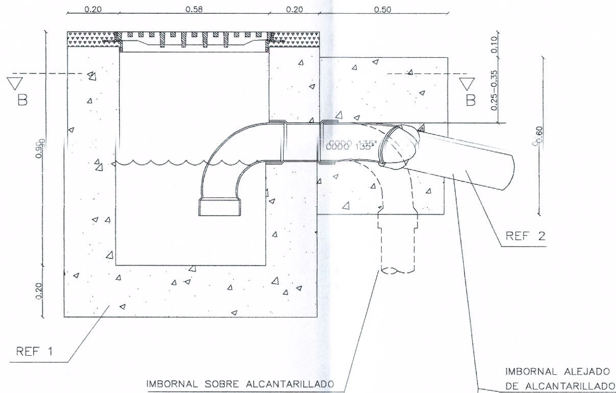
SECCION A-A
