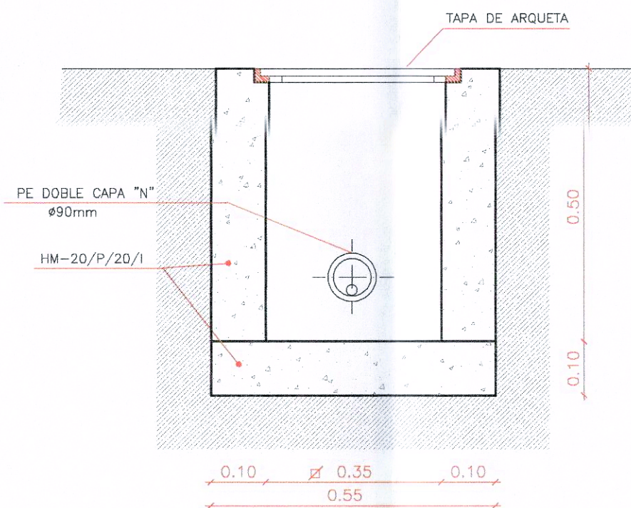
ARQUETA DE PASO O REGISTRO
