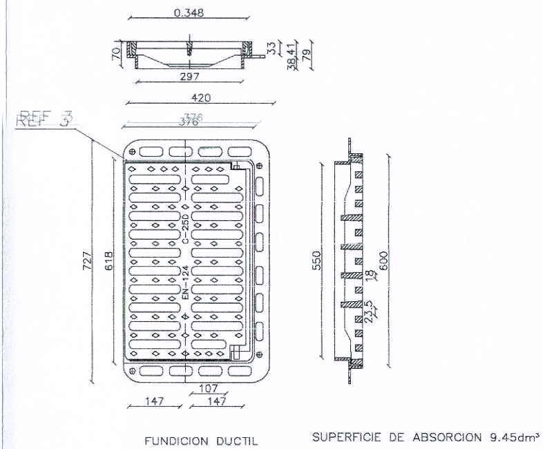
REJA ABATIBLE CON MARCO
