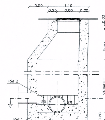
ALZADO
