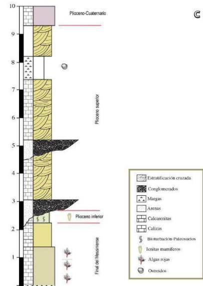
2. ESQUEMA GEOLÓGICO.
